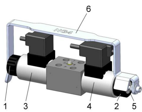
Wegeventil NG4
